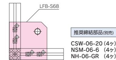
M6シリーズ取付例
