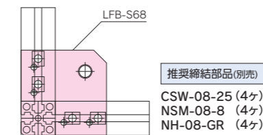
M8シリーズ取付例
