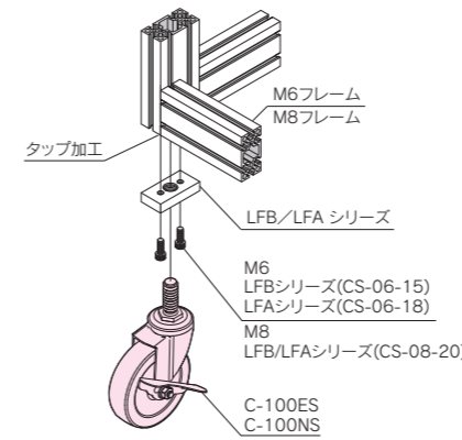
■ キャスター 取付例 ※厚さ4mm以下の薄型スパナ(サイズ23)をご使用下さい。
