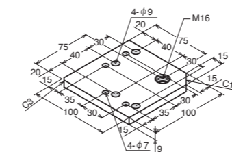
M8シリーズ取付例
