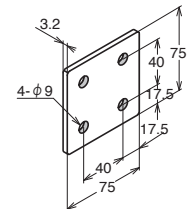
BPSM-7575-8
