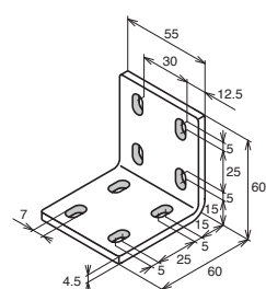
BLHL-5560-6
