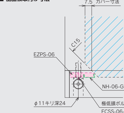
■樹脂板取り付け寸法
