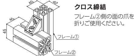
フラット面取付 フラット面締結側の爪を折りご使用ください。
