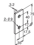
BPSM-3575-8
