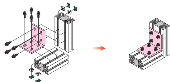
NSM-06-6 + NH-06 締結ボルト
