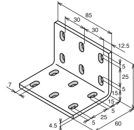
BLHL-8560-6
