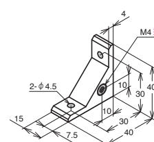
ABCH-4015-4
