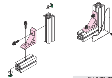
パネル取付例
