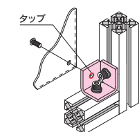
パネル取付例
