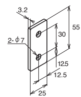
BPSM-2555-6
