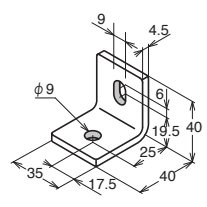
BLSM-4035-8
