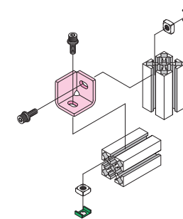
パネル取付例
